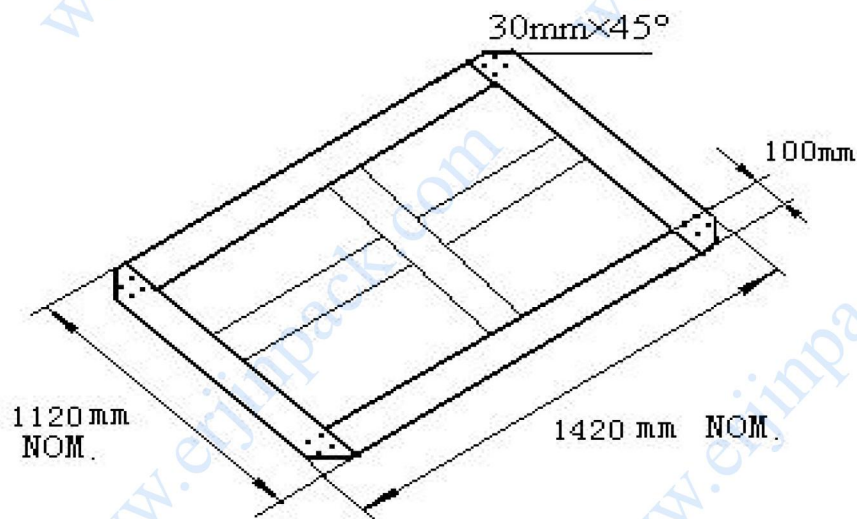
TOP FRAME 顶板
