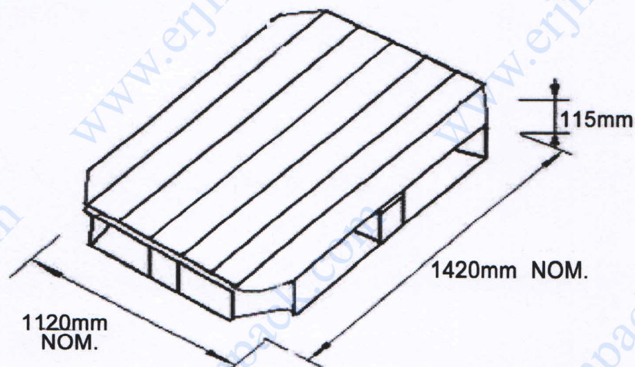
4-WAY PALLET 卡板
