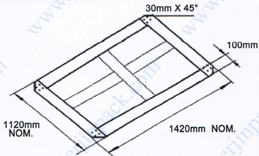
TOP FRAME 顶板
